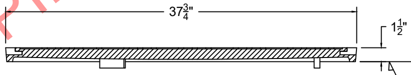
SECTION A-A
